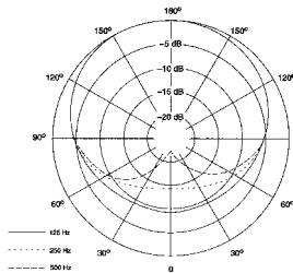
TYPISCHE RICHTCHARAKTERISTIK
