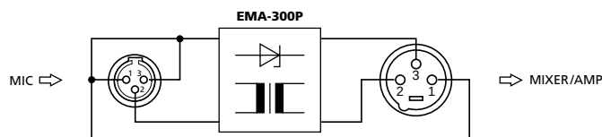
Beschlutung • Circuit diagram • Schéma électrique • Schema elettrico
